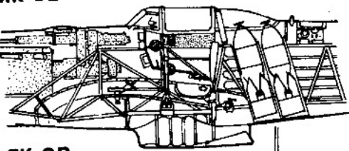
ЯК-9Р
